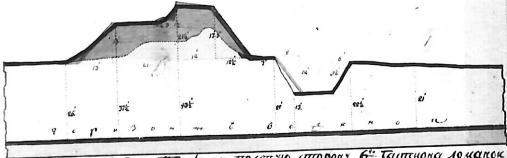
До 21. Профиль полевой стороны 6-го таптика ложакоб къртылы.
