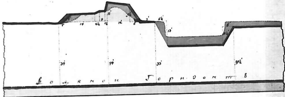
До 12. Профиль лепого фазу 3-го таптика.
