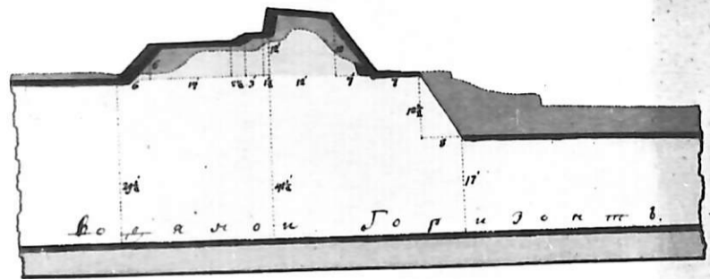
До 7. Профиль пракои стороны каръжкоб полигона къртылы.
